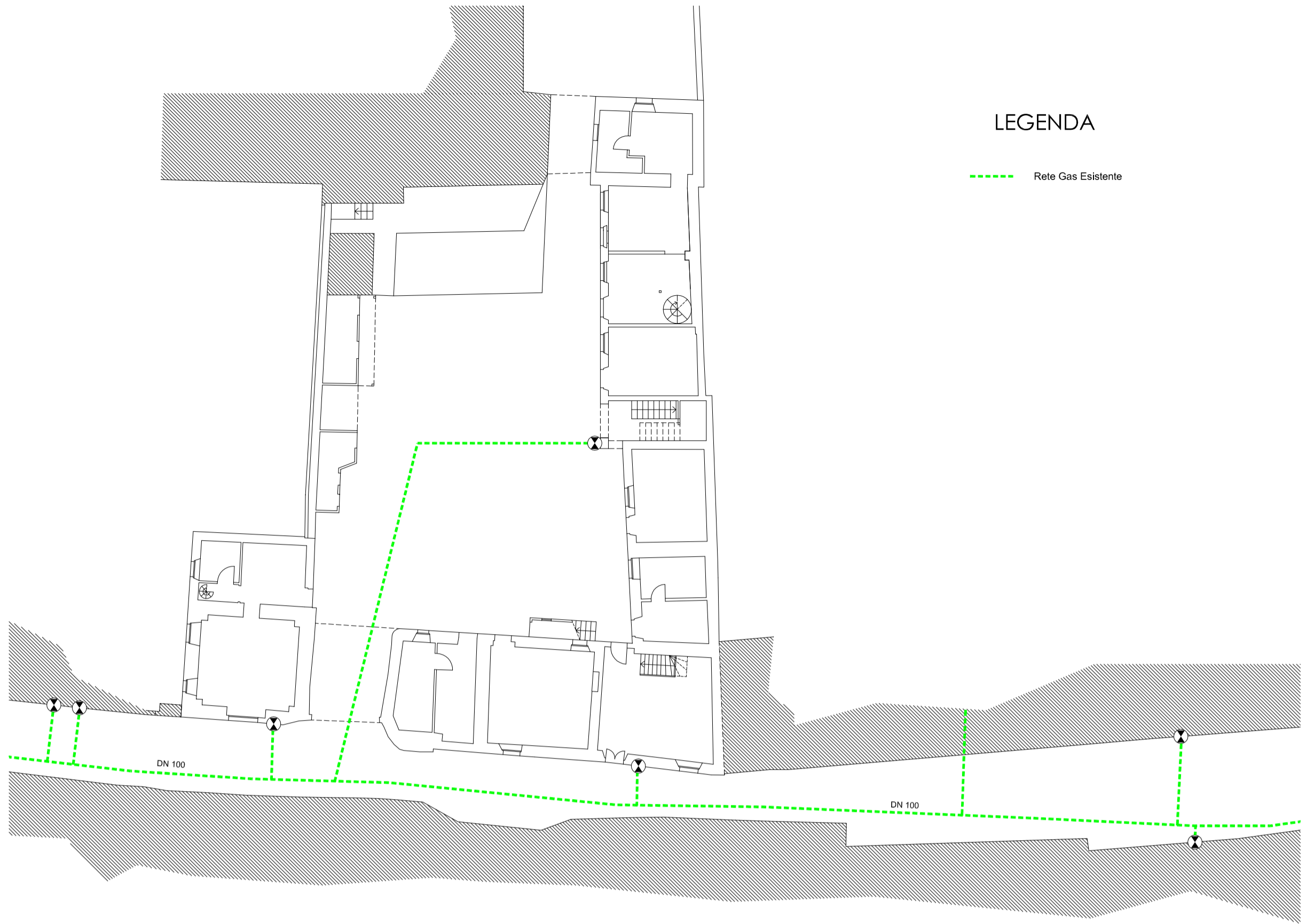
Stato di fatto Schema rete gas metano scala 1:200
