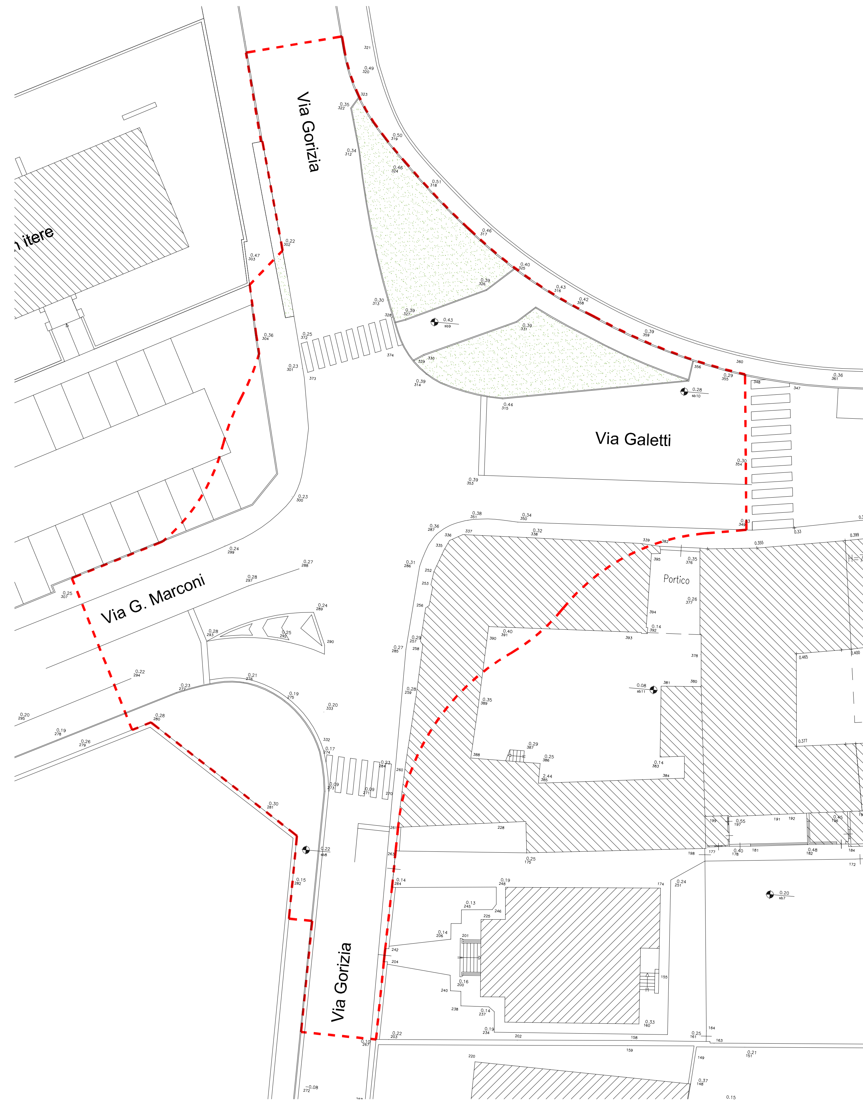
PLANIMETRIA AREA DI INTERVENTO STATO DI FATTO
