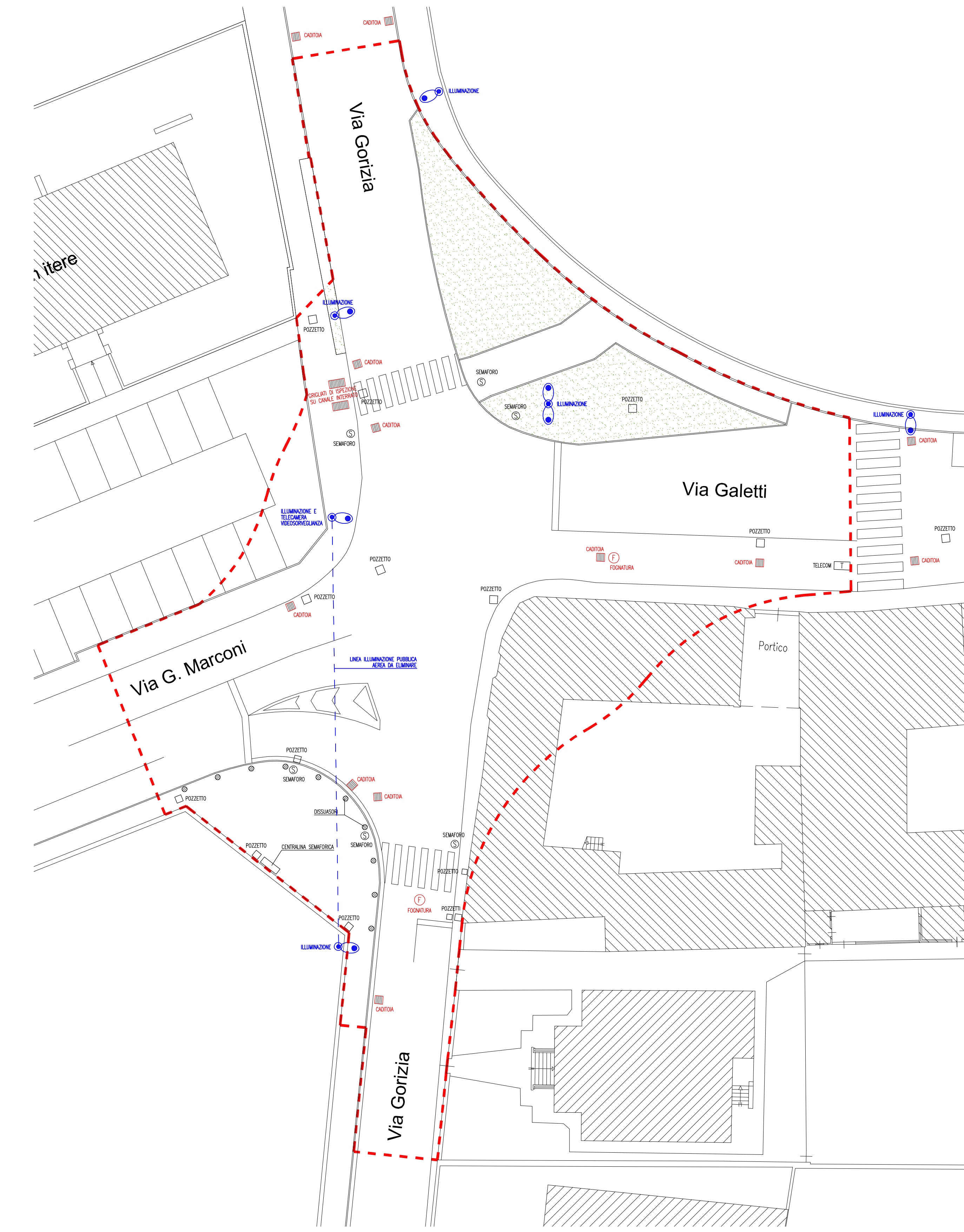
PLANIMETRIA IMPIANTI ILLUMINAZIONE PUBBLICA E SMALTIMENTO ACQUE STATO DI FATTO
