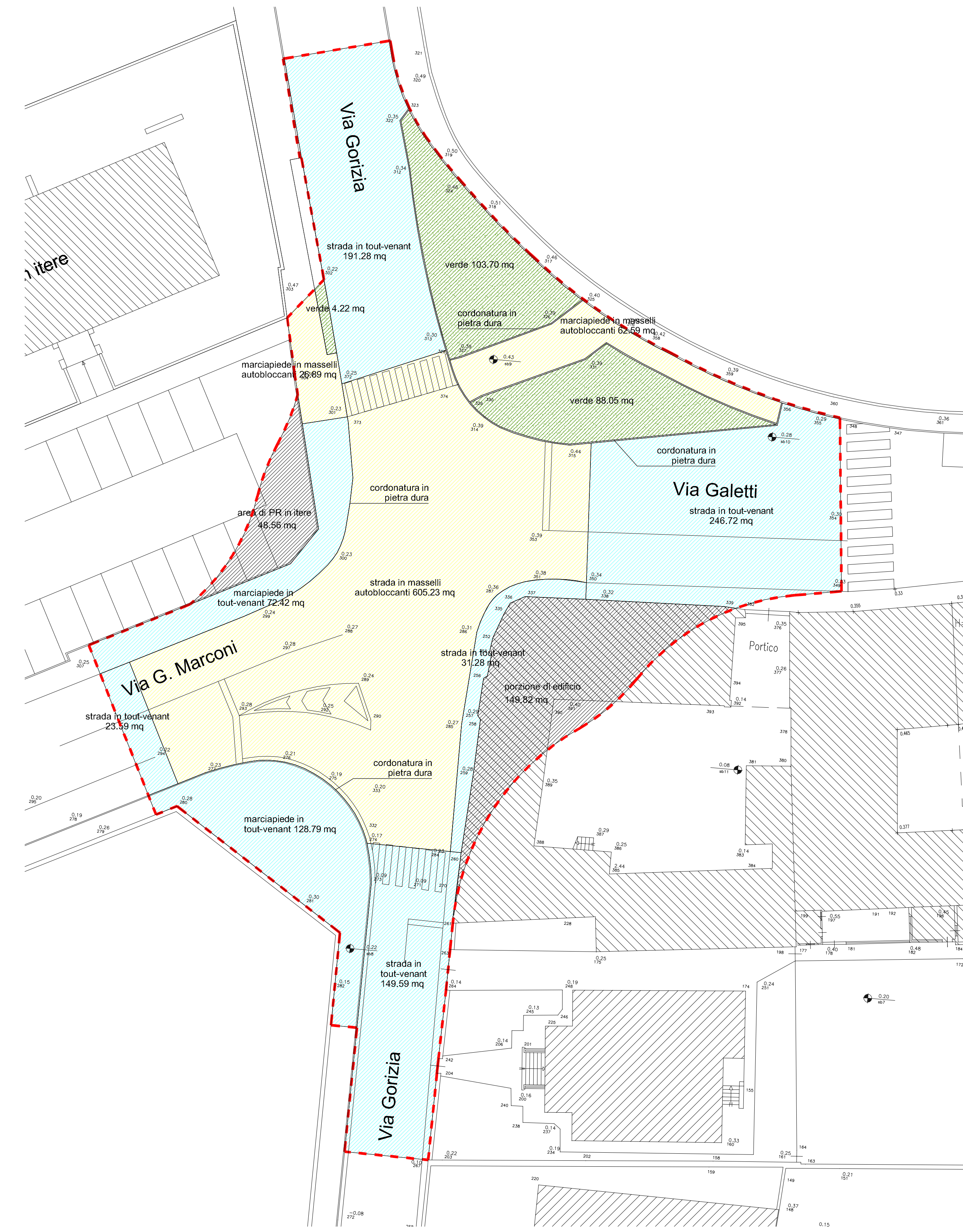
PLANIMETRIA FINITURE SUPERFICIALI STATO DI FATTO
