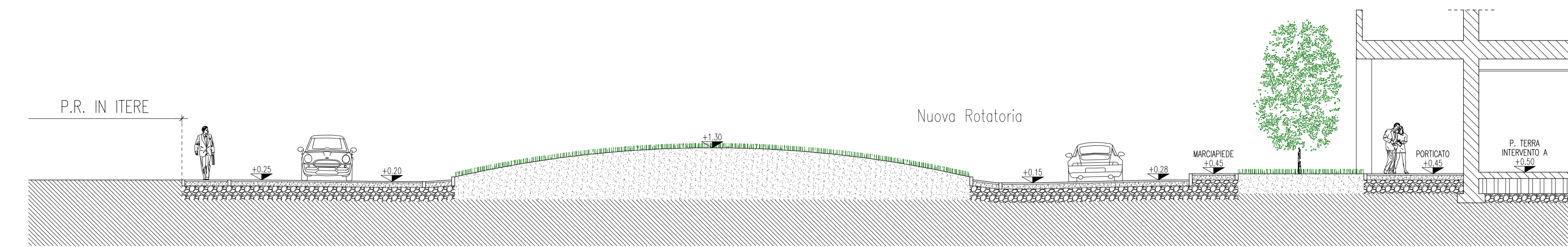
SEZIONE R2-R2
