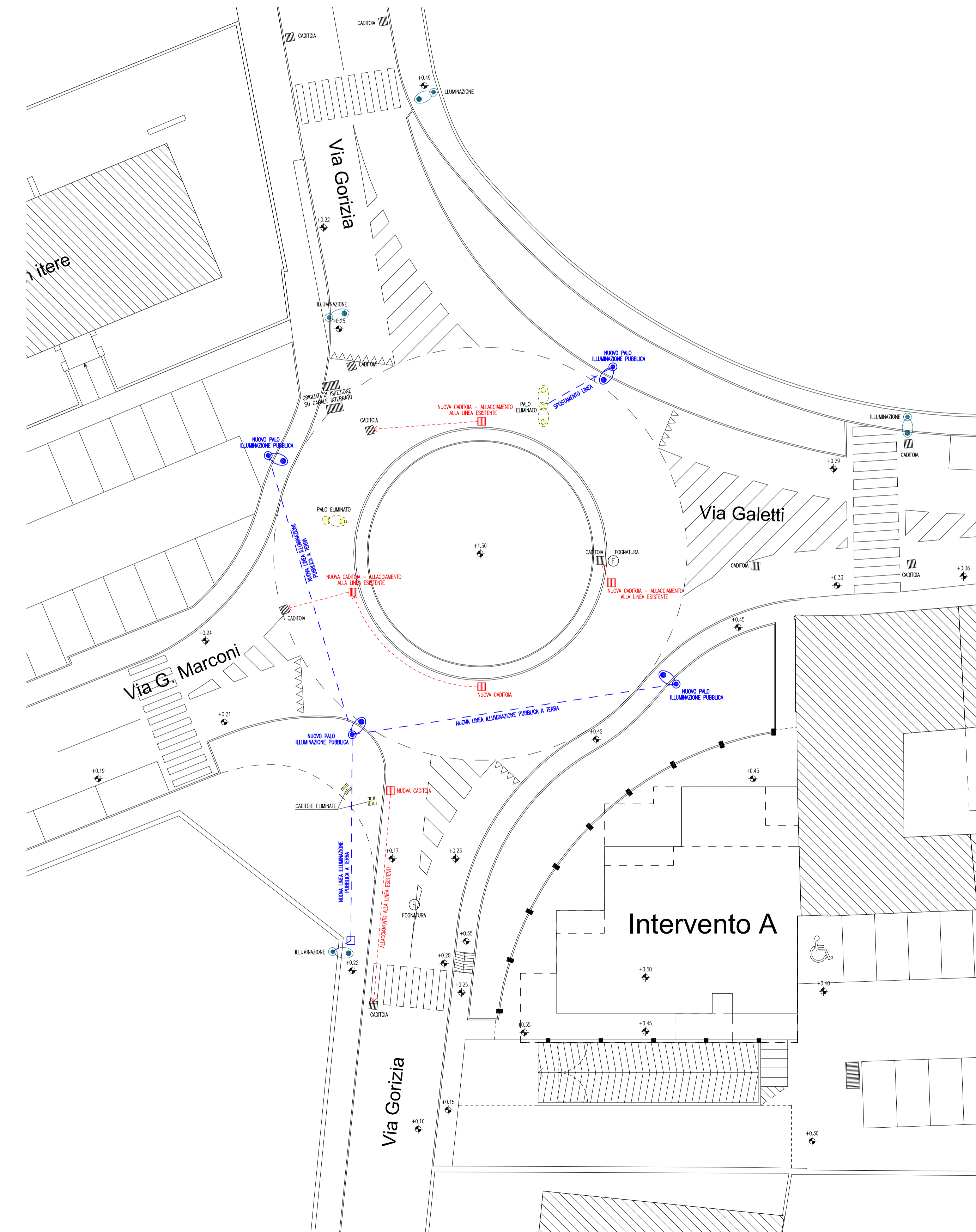
PLANIMETRIA IMPIANTI ILLUMINAZIONE PUBBLICA E SMALTIMENTO ACQUE PROGETTO
