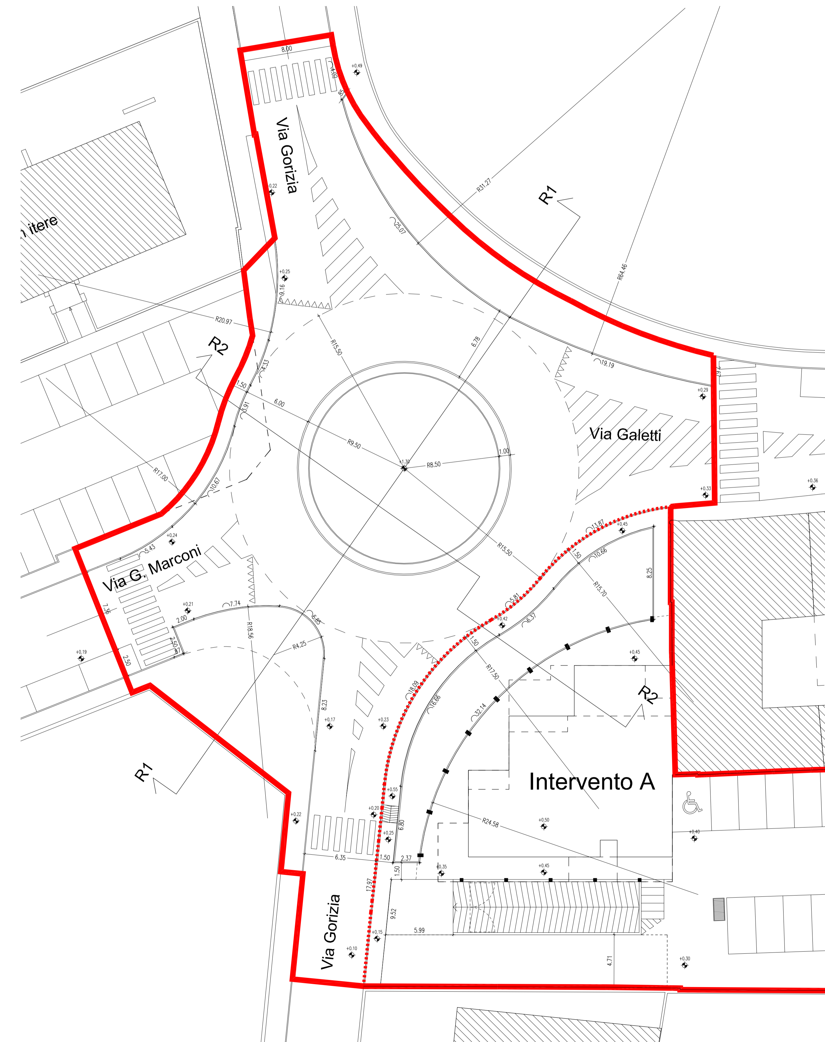
PLANIMETRIA AREA DI INTERVENTO PROGETTO
