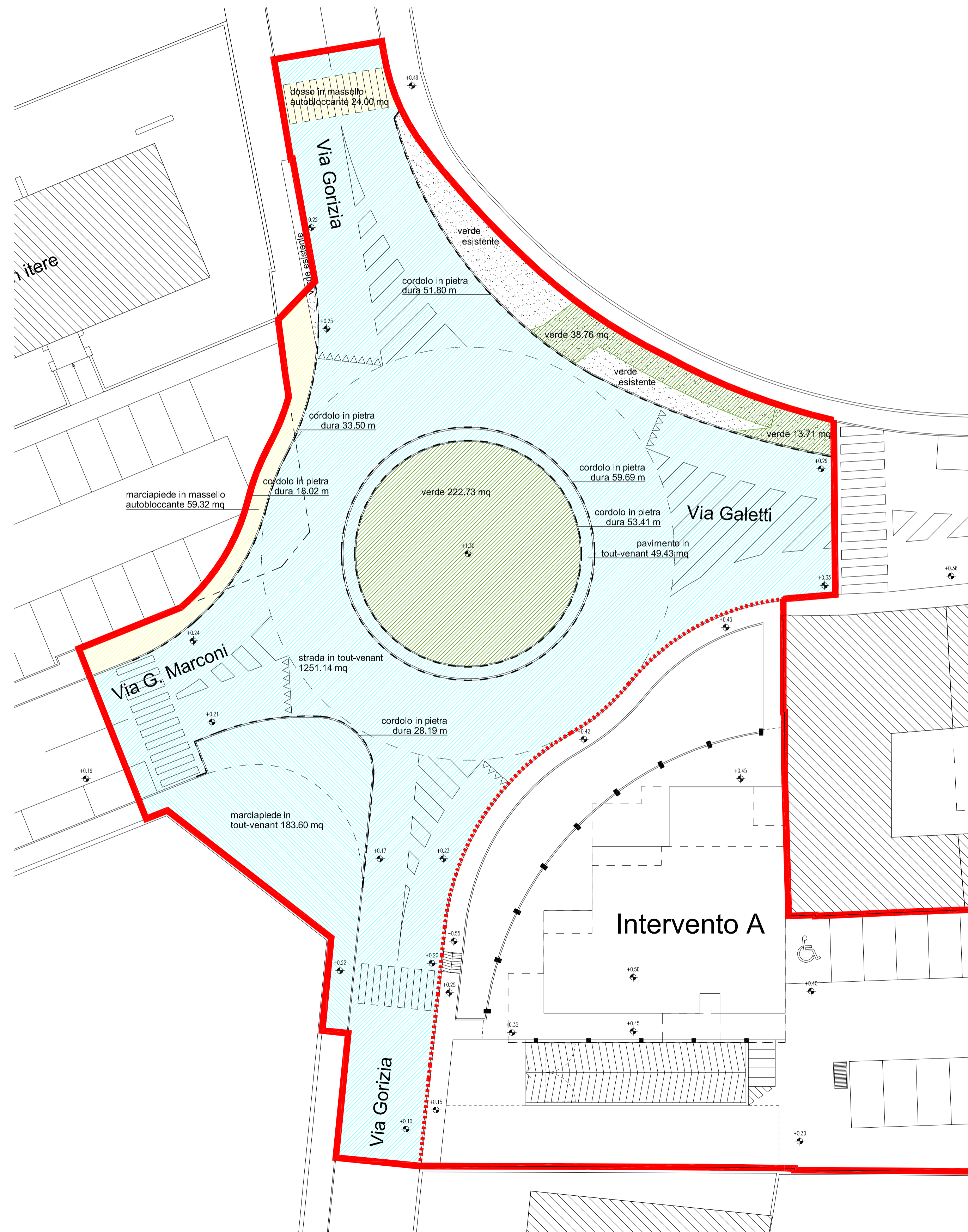
PLANIMETRIA FINITURE SUPERFICIALI PROGETTO
